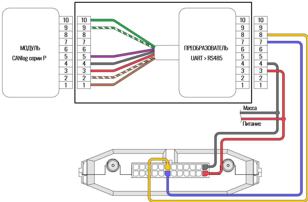
Рисунок 2.24 Подключение CAN-LOG через переходник UART-RS485
