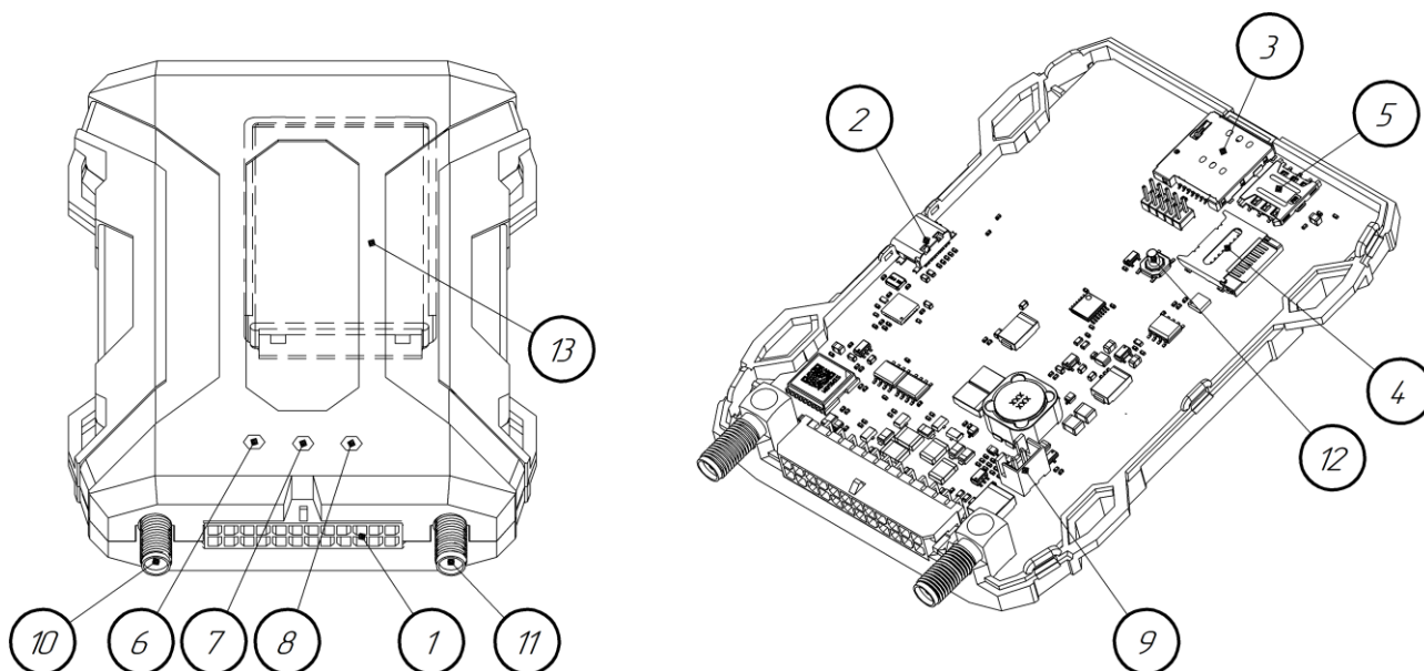
Рисунок 2.1 Основные элементы
