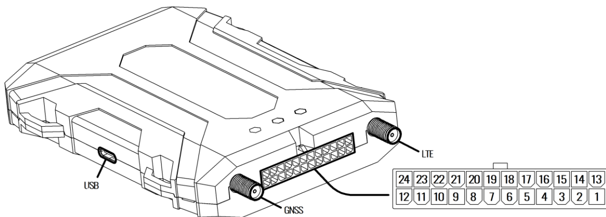
Рисунок 2.2 Нумерация выводов
