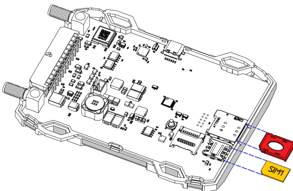
Рисунок 2.4 Установка SIM-карт
