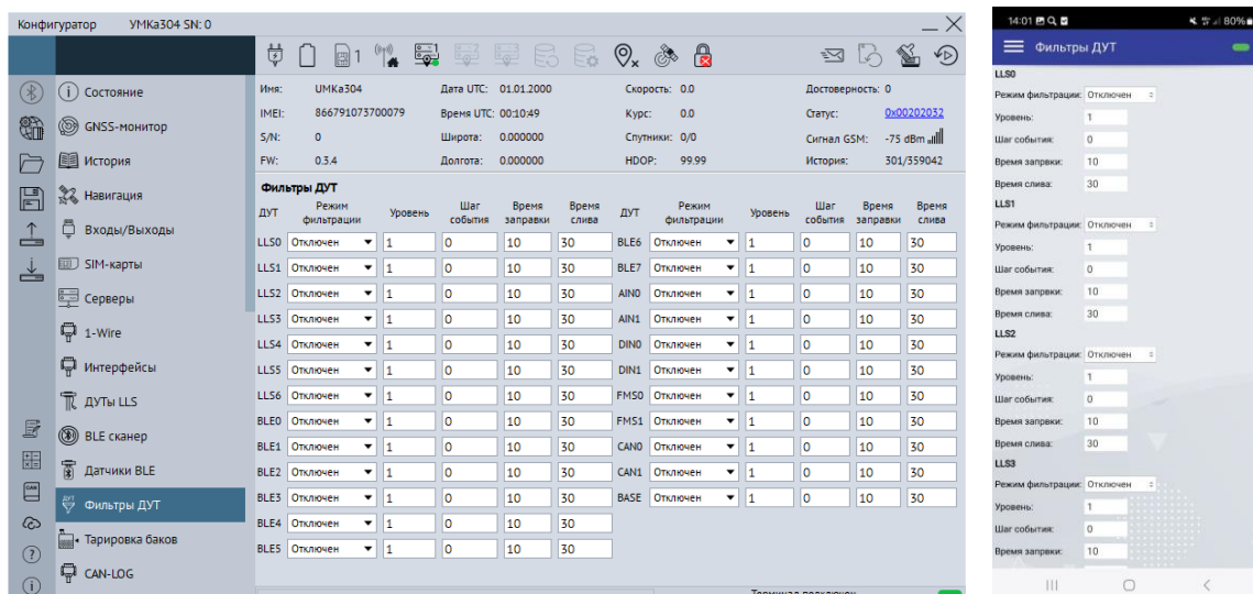
Рисунок 3.28 Вкладка «Фильтры ДУТ»
