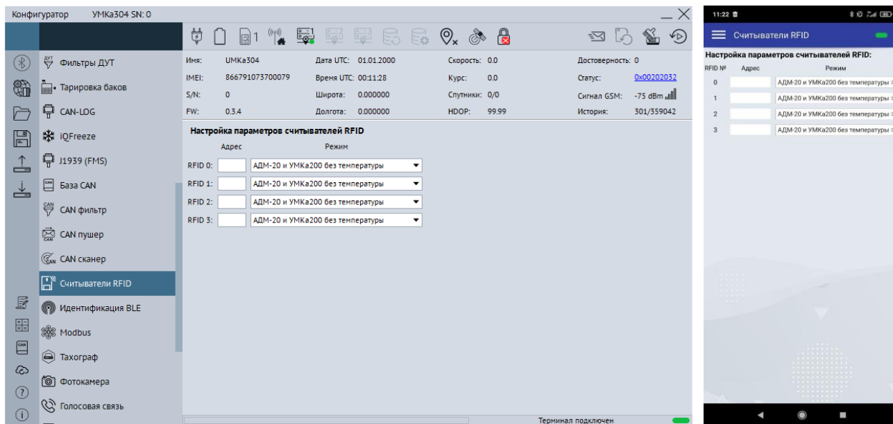
Рисунок 3.39 Вкладка «Считыватель RFID»
