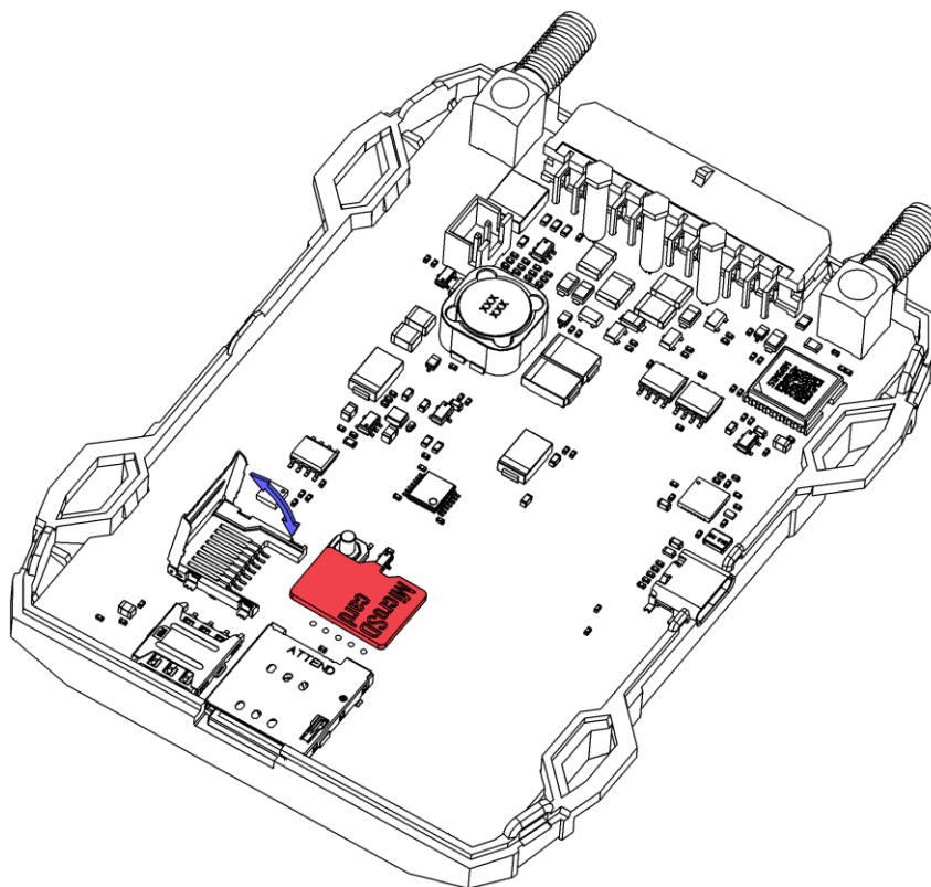
Рисунок 2.6 Установка microSD-карты
