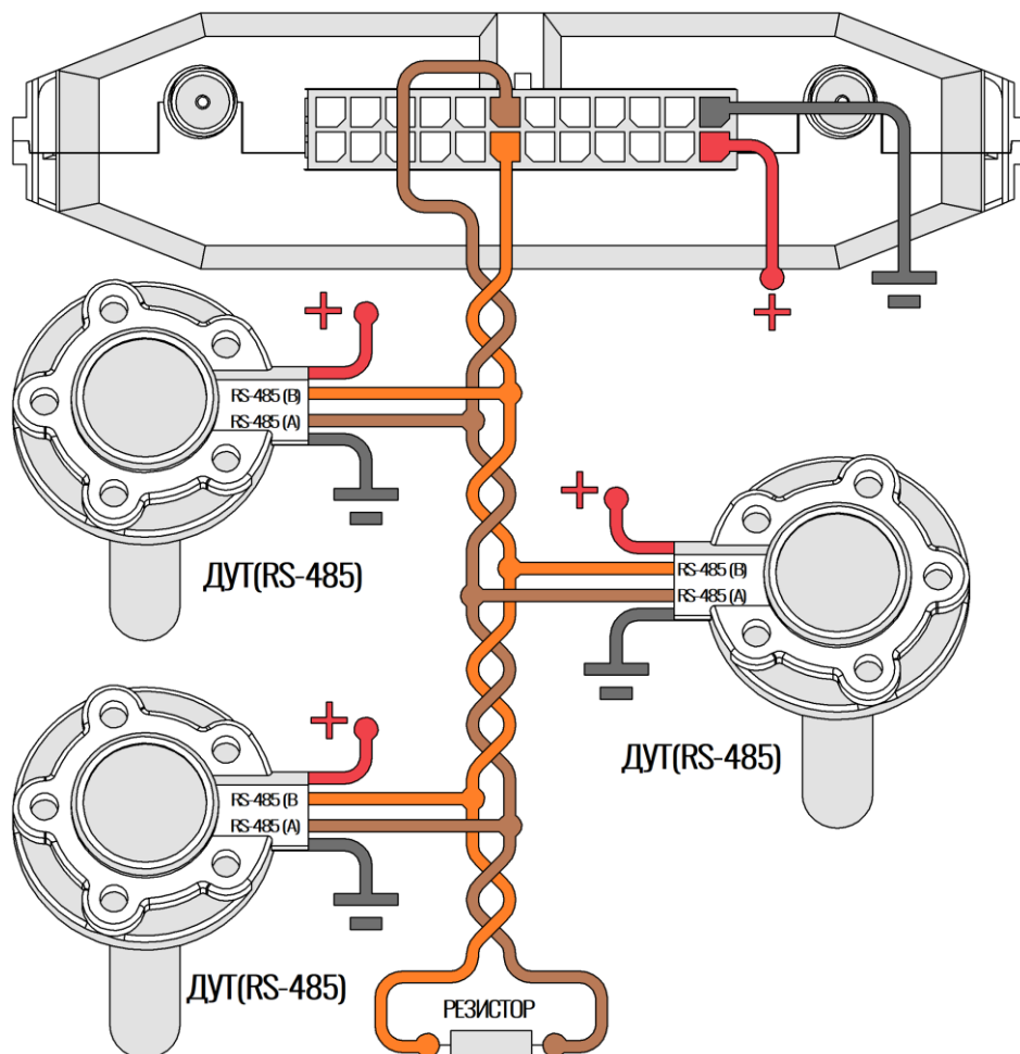
Рисунок 2.17 Подключение ДУТ по интерфейсу RS-485
