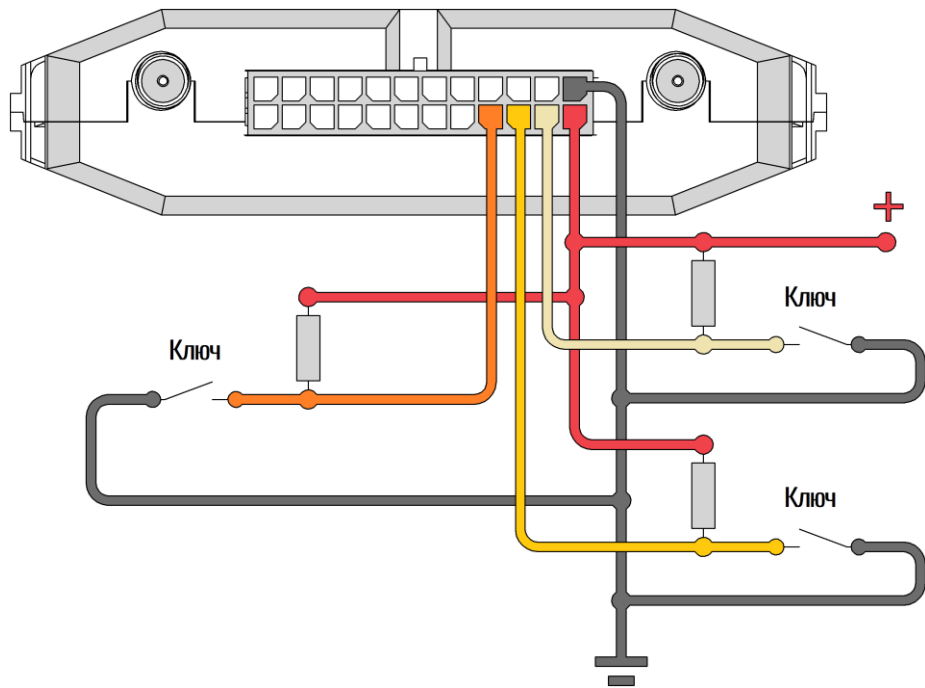
Рисунок 2.9 Подключение с подтяжкой к «+»
