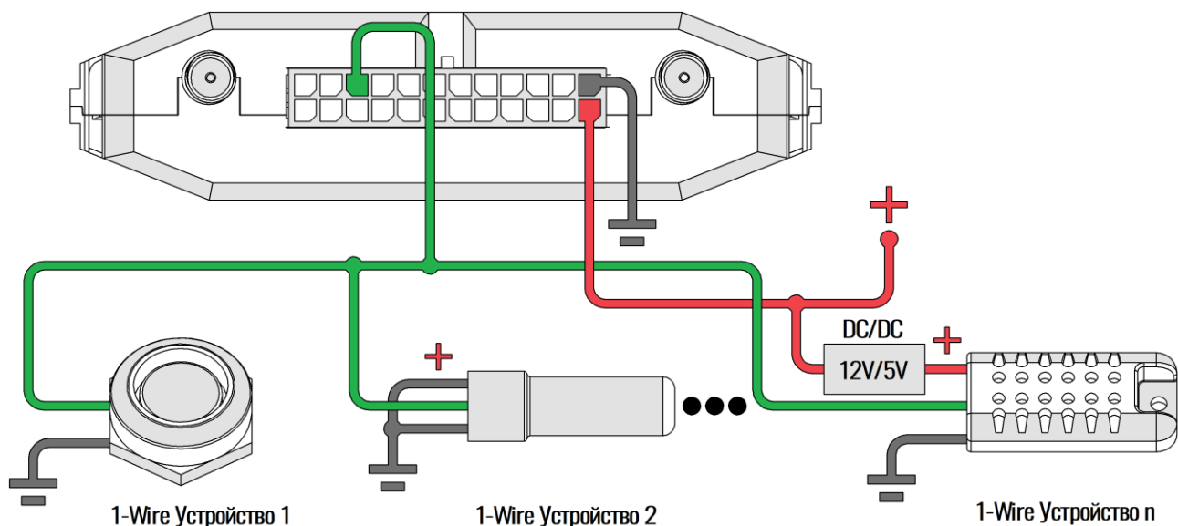
Рисунок 2.22 Подключение устройств по 1-Wire
