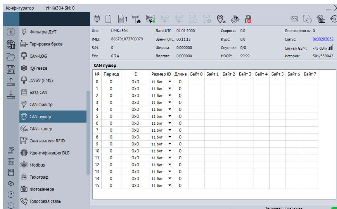
Рисунок 3.37 Вкладка «CAN пушер»
