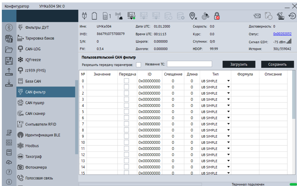
Рисунок 3.36 Вкладка «CAN фильтр»
