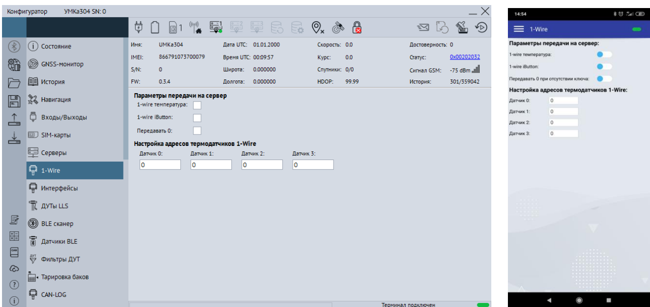
Рисунок 3.22 Вкладка «1-Wire»
