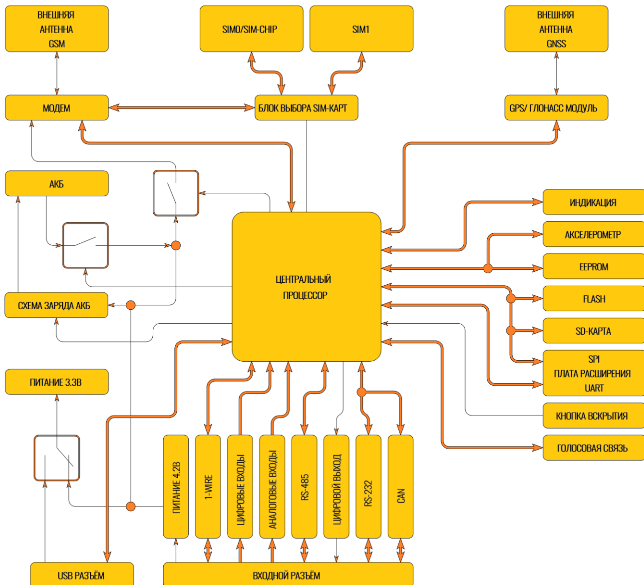
Рисунок 1.3 Блок-схема АСН 304
