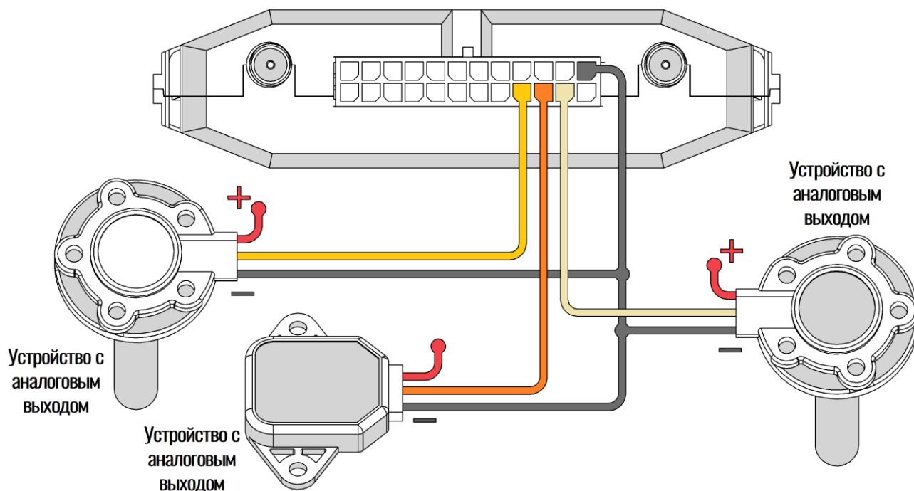
Рисунок 2.8 Подключение аналоговых источников
