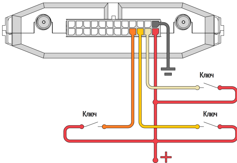
Рисунок 2.10 Подключение с подтяжкой к «-»
