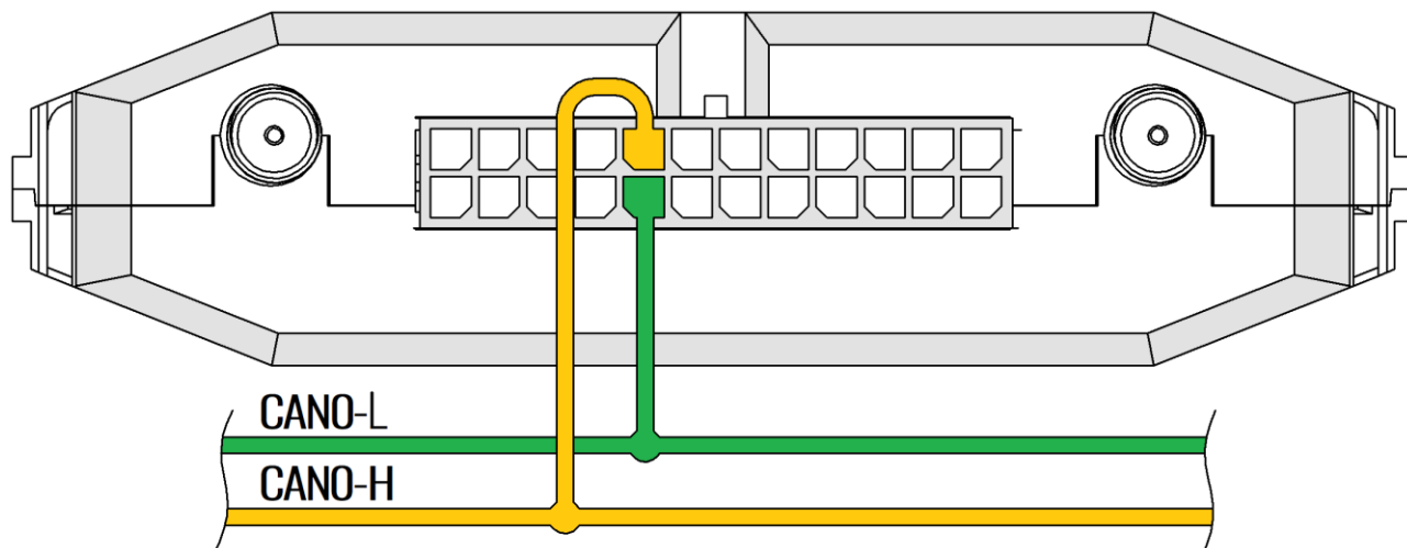
Рисунок 2.20 Подключение к шине CAN
