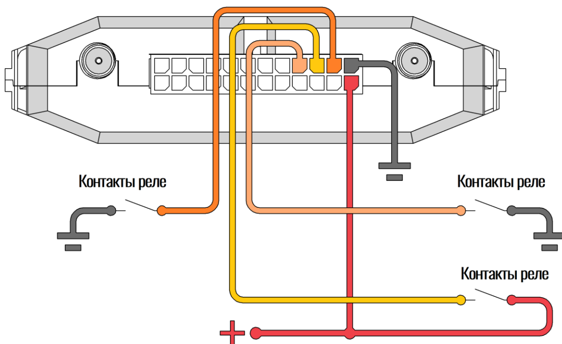
Рисунок 2.12 Варианты подключения дискретных датчиков
