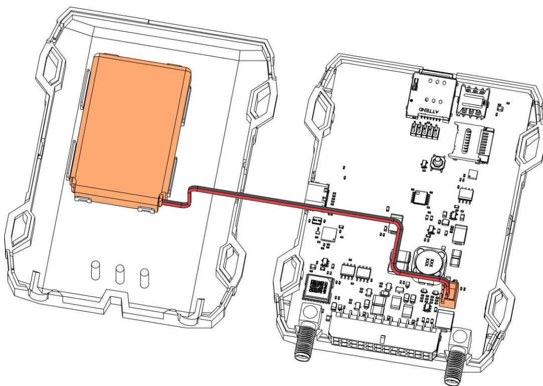
Рисунок 2.5 Установка аккумулятора
