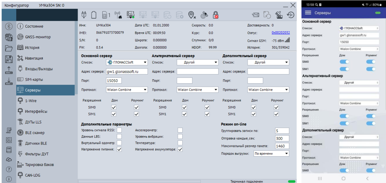
Рисунок 3.21 Вкладка «Серверы»
