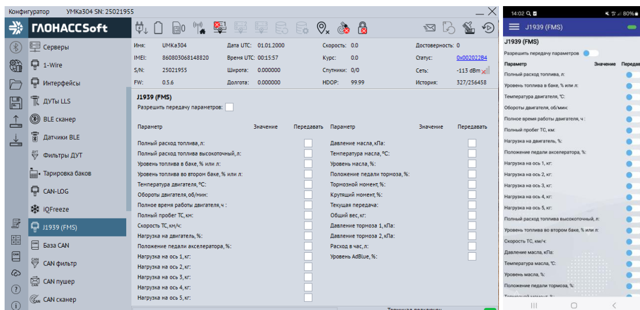
Рисунок 3.33 Вкладка «J1939(FMS)»
