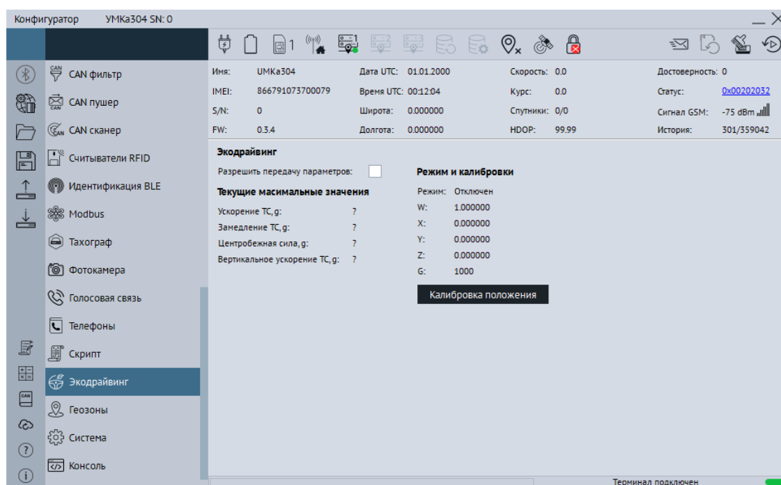
Рисунок 3.49 Вкладка «Экодрайвинг»
