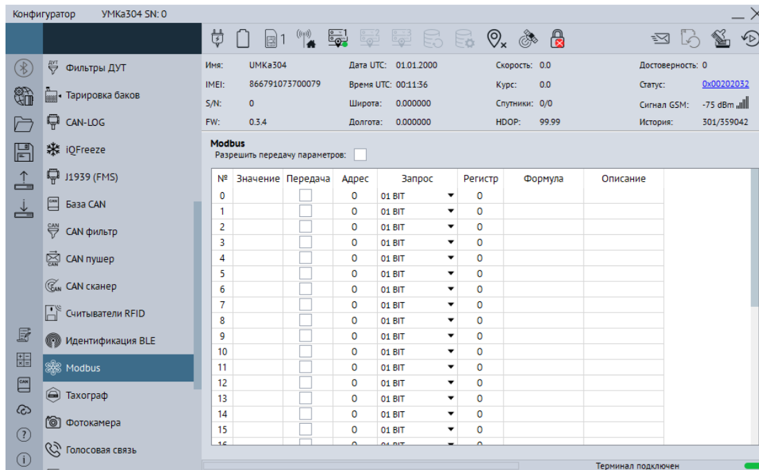
Рисунок 3.41 Вкладка «Modbus»
