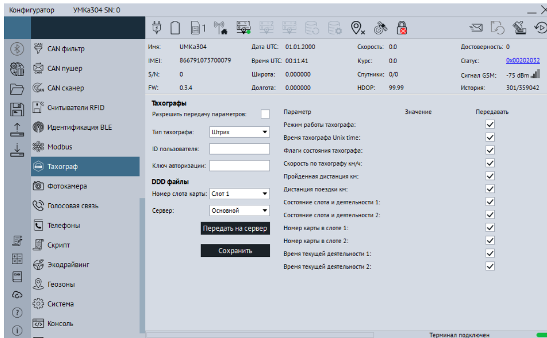
Рисунок 3.42 Вкладка «Тахографы»
