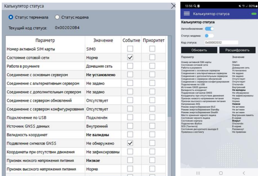
Рисунок 3.14 Калькулятор статуса
