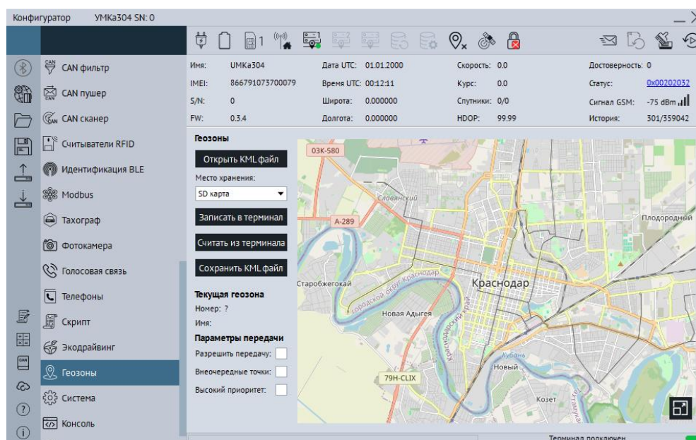
Рисунок 3.51 Вкладка «Геозоны»
