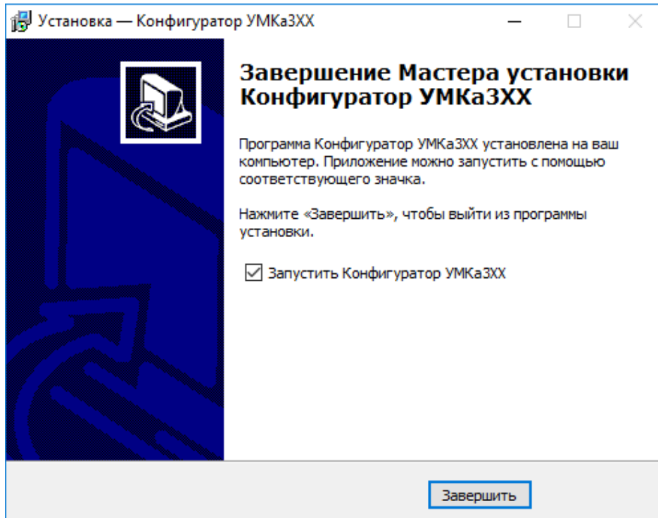
Рисунок 3.7 Запуск приложения
